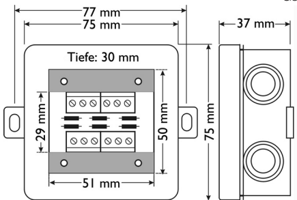
Massbilder G3
