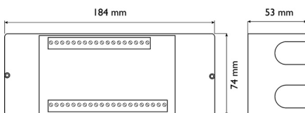
G6 Auf-/Unterputzmontage
